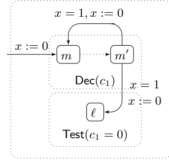
Fig. 9. Module \text{Test}(c_1 > 0)
