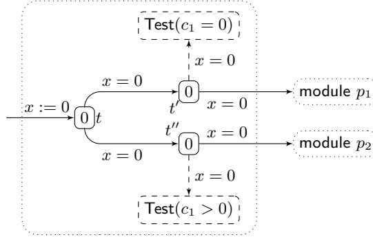
Fig. 10. Module \text{Cond}(c_1 = 0)
