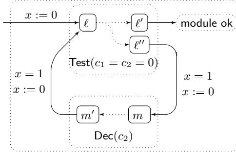
Fig. 8. Module \text{Test}(c_1 = 0)
