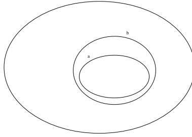
FIG. 5 – cas où n(a) = 1296 , n(b) = 2304 , n(a \wedge b) = 1296
