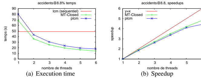
FIG. 1 – Résultats pour accidents à 8.8% (dense)
